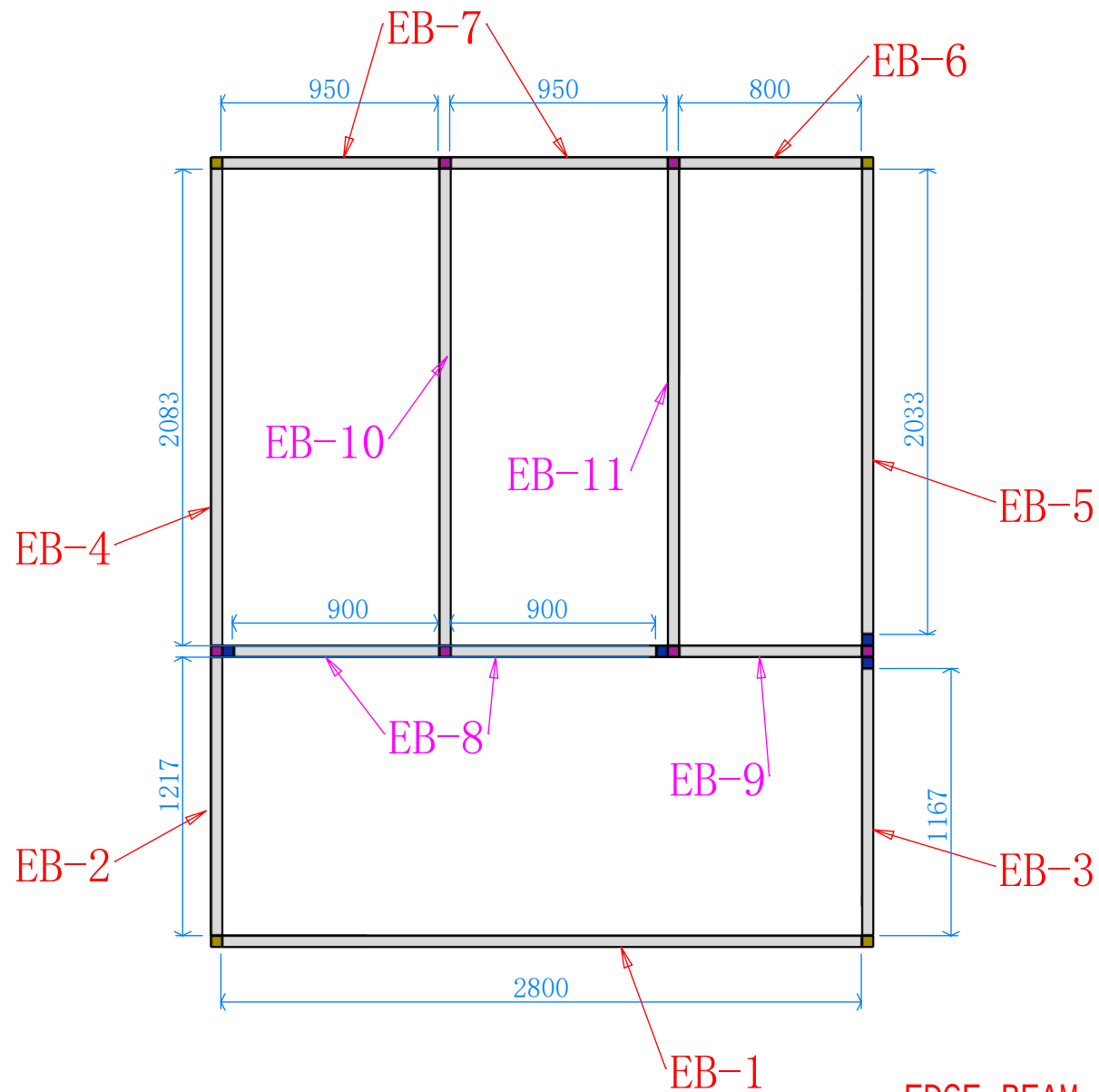
EDGE BEAM ASSEMBLY
